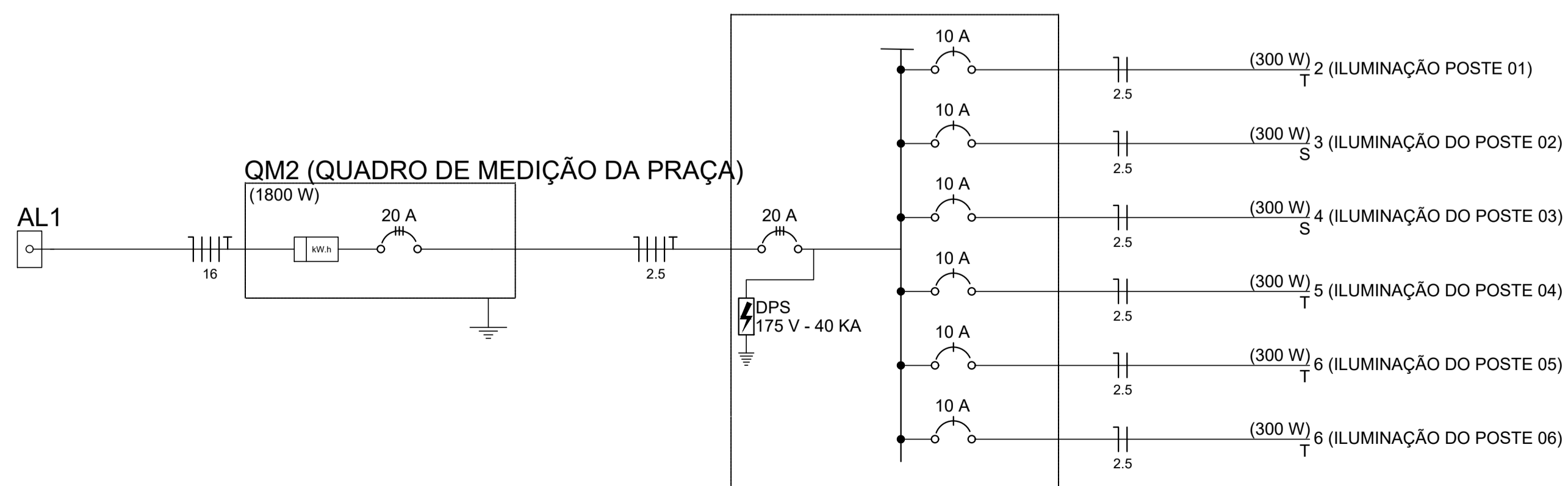
QD1 (QUADRO DE DISTRIBUIÇÃO DA PRAÇA) (6024 W)
