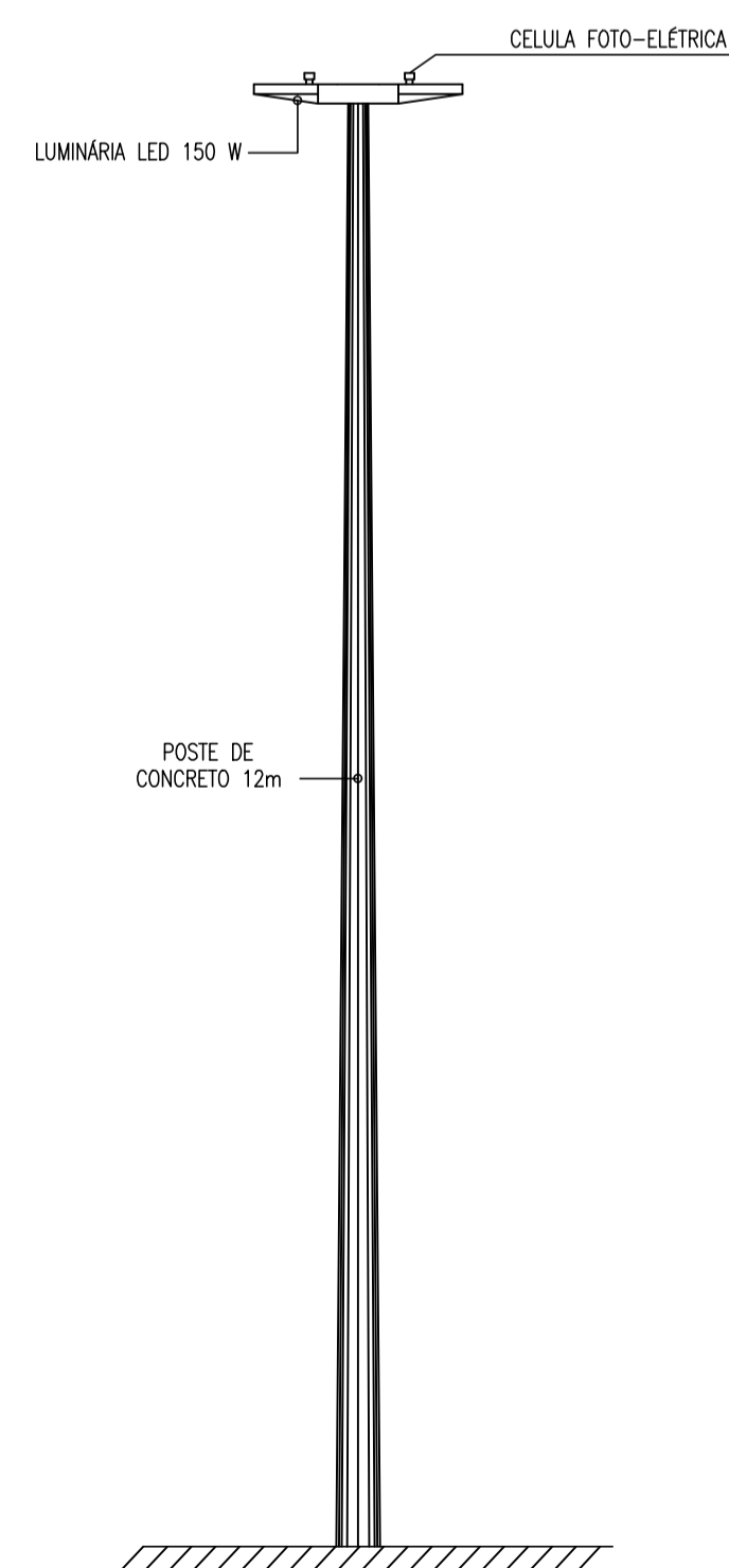
VISTA FRONTAL ESCALA 1/50
