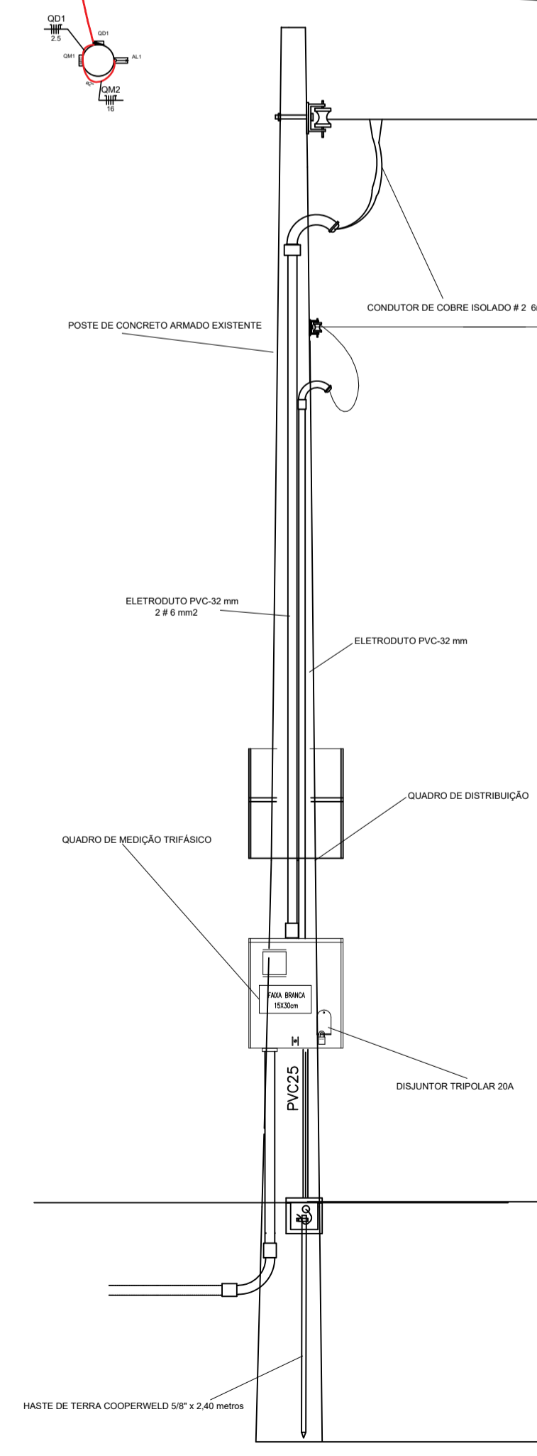
DET - POSTE DE ENTRADA DE ENERGIA ESCALA 1/125
