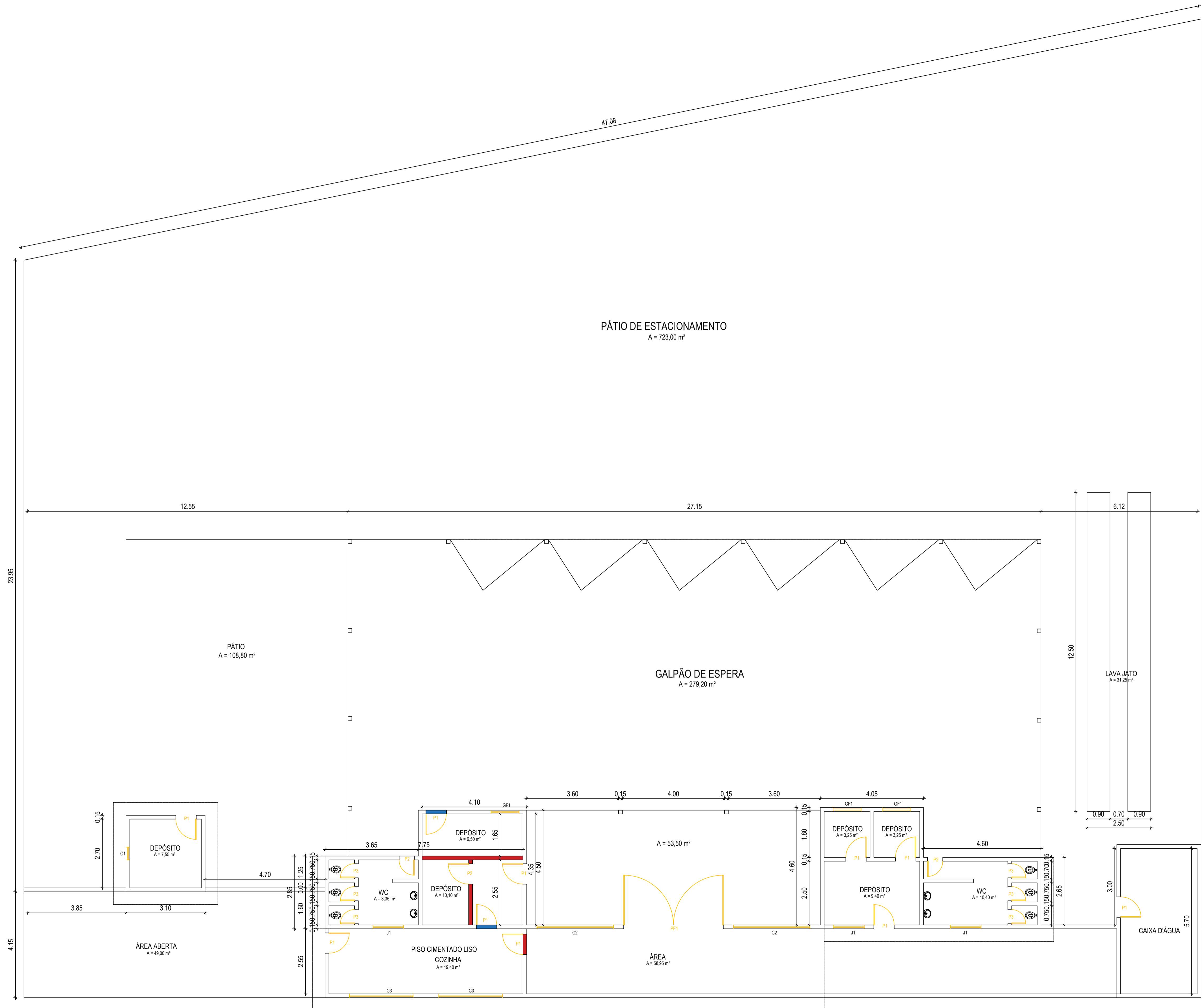
1 PLANTA BAIXA EXISTENTE ESCALA 1:100
