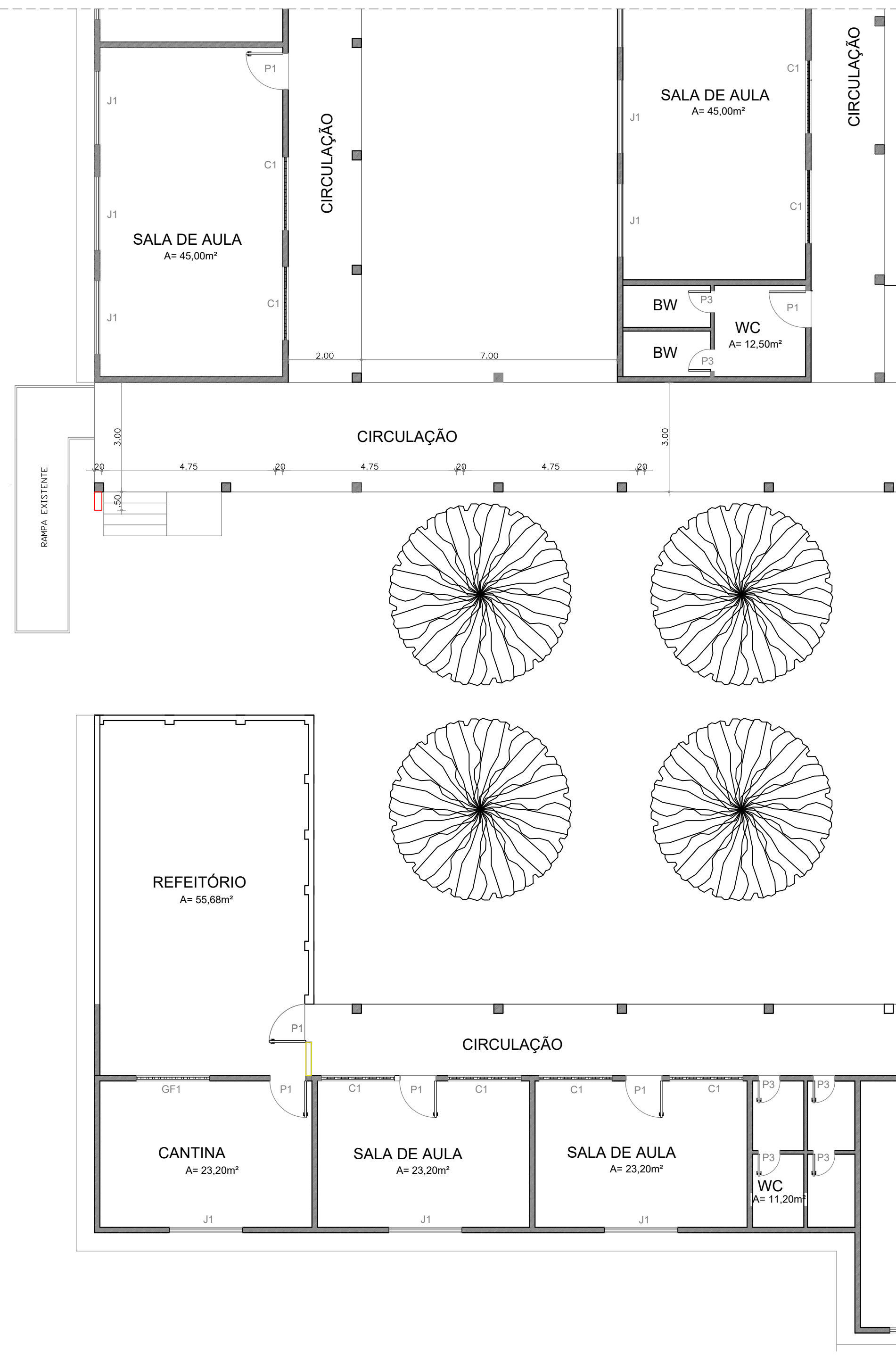
1 PLANTA DE LEVANTAMENTO ESCALA 1:100
