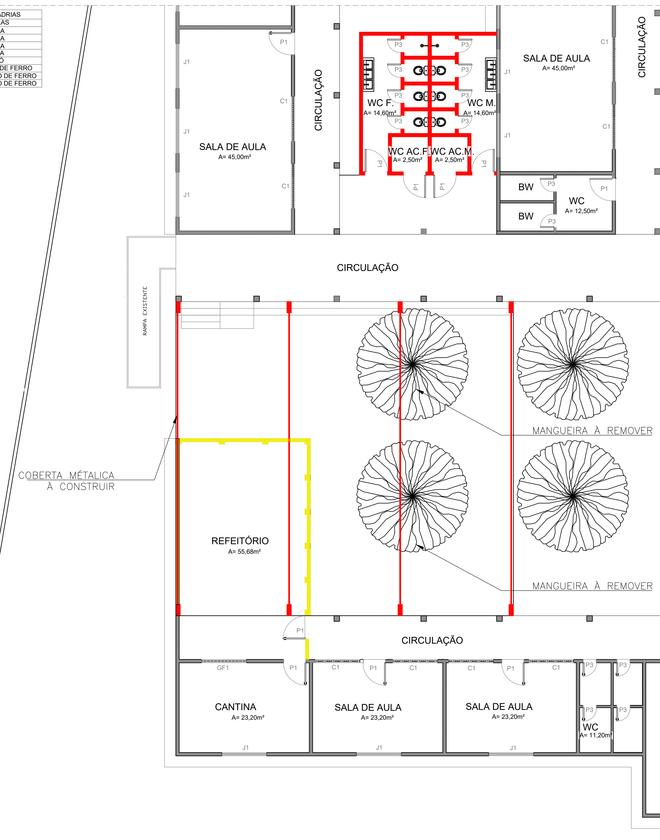
2 PLANTA DE CONSTRUIR/DEMOLIR ESCALA 1:100
